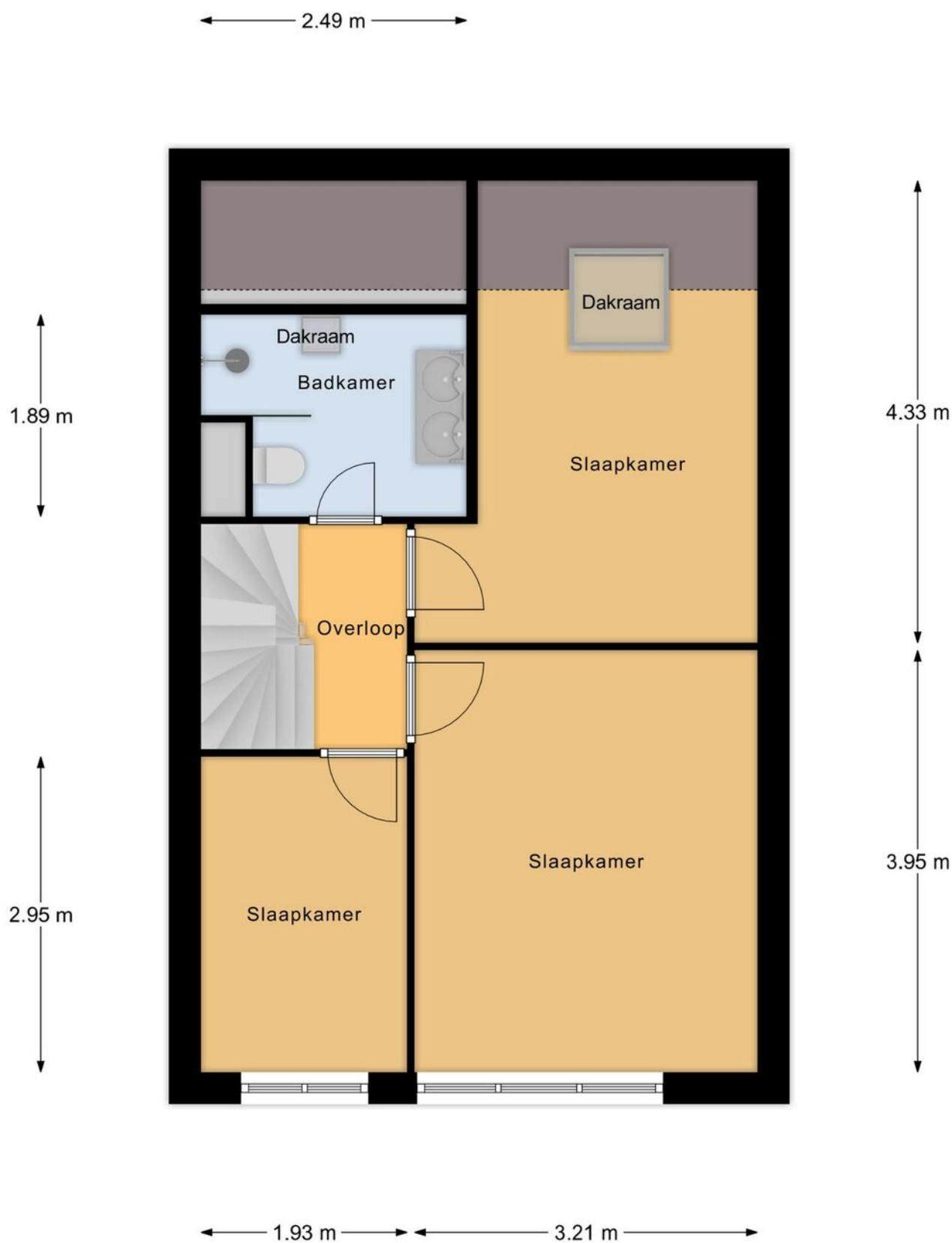
1e Verdieping
